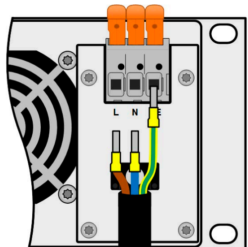
Bild 10 - Beispielkonfiguration eines AC-Kabels
