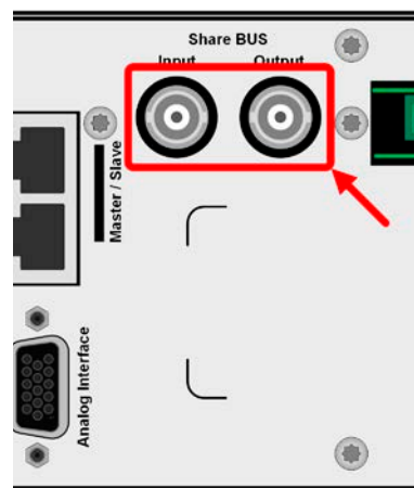
Bild 5 - Share-Bus
