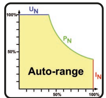
Bild 14 - Leistungsfläche
