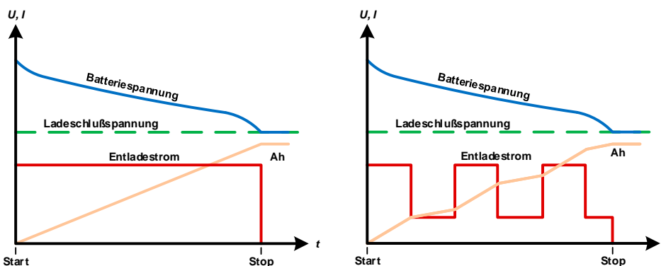
Statische Entladung
