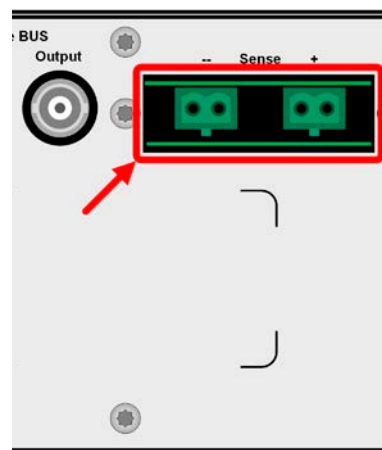
Bild 6 - Fernfühlungsanschlüsse
